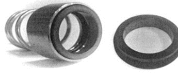
TIPO: T5SD-V DIN 24960
